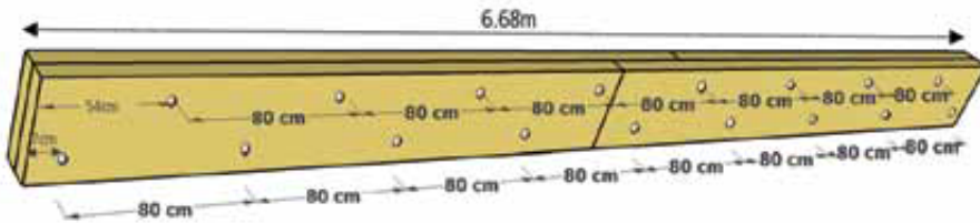
Ubicación de los clavos para la unión de la viga cunbrera
