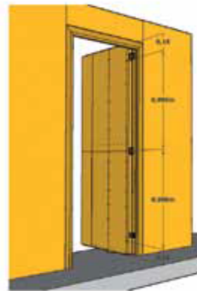
Distancia entre colocación de bisagras ejes
