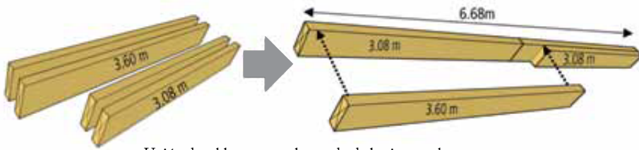
Unión de tablon para el armado de la viga cunbrera
