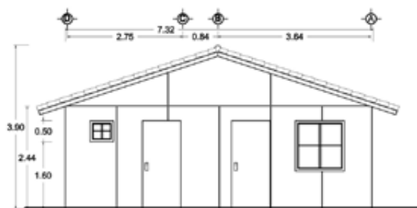
Fachada laterales
