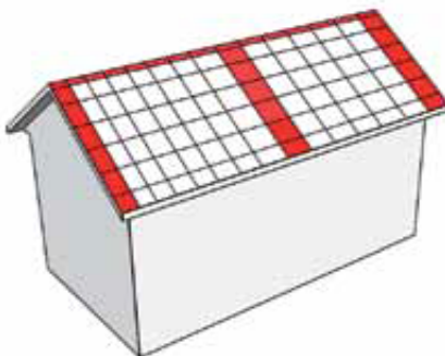
Tejas pegadas con mortero
