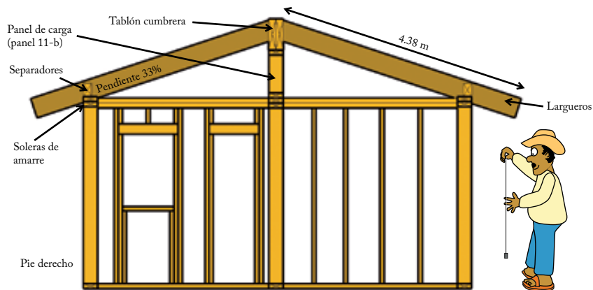
Techos de largueros sobre tablón cumbreira
