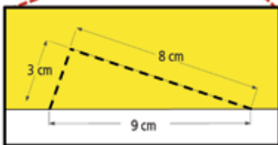
Unión de larguero a panel
