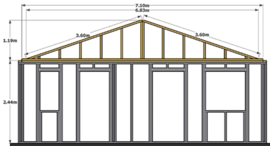
Panel tímpano para techo de largueros
