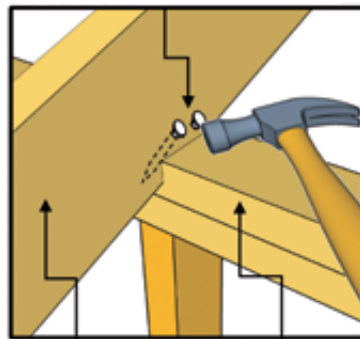
Larguero
