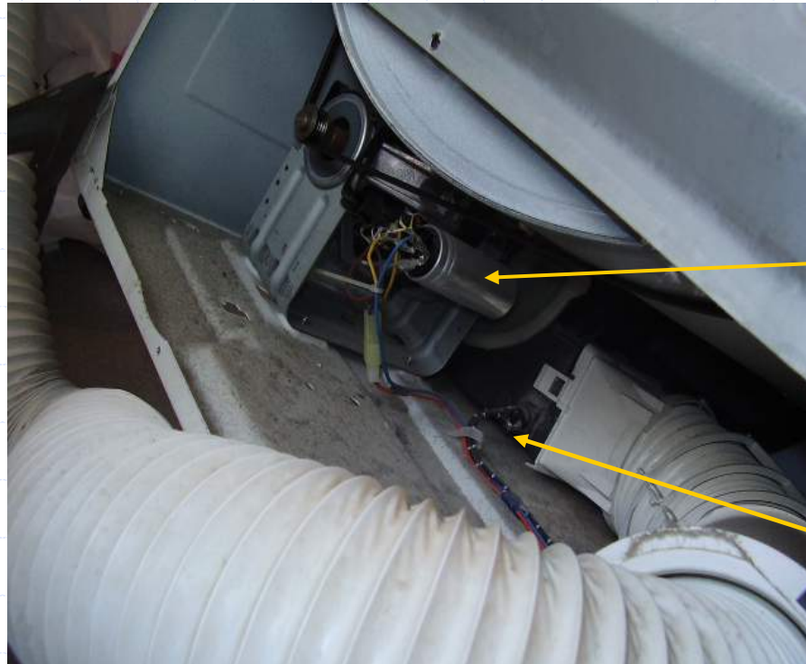
Condensador
