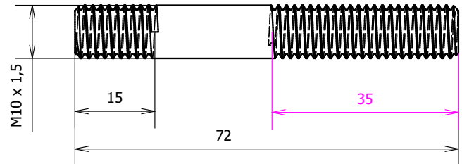
G-G ( 1 : 1 )
