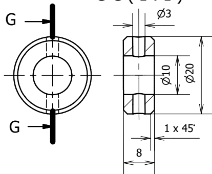
G-G ( 1 : 1 )
